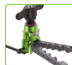
Listwa rozszerzająca jest włożona do korpusu
